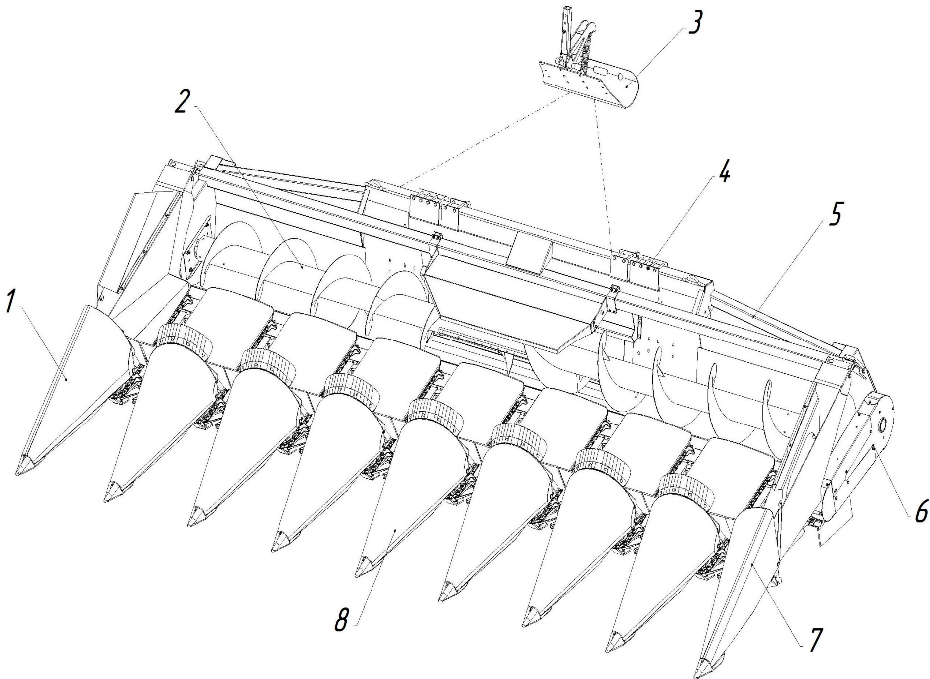
Рисунок Рис.1 Общий вид жатки ЖК-82.00.000
