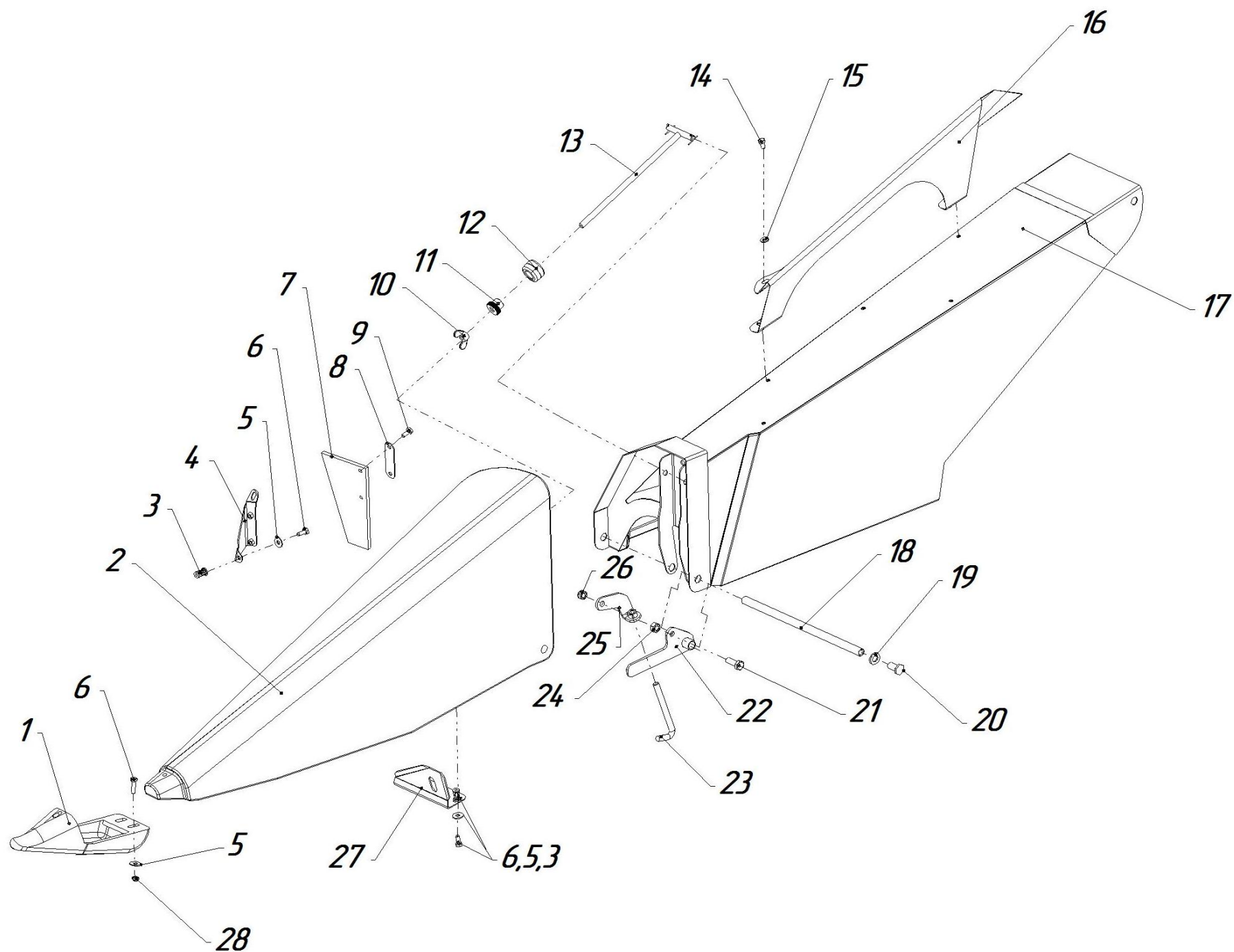
Рисунок 31 Делитель ЖК- 82.09.000(-01)
