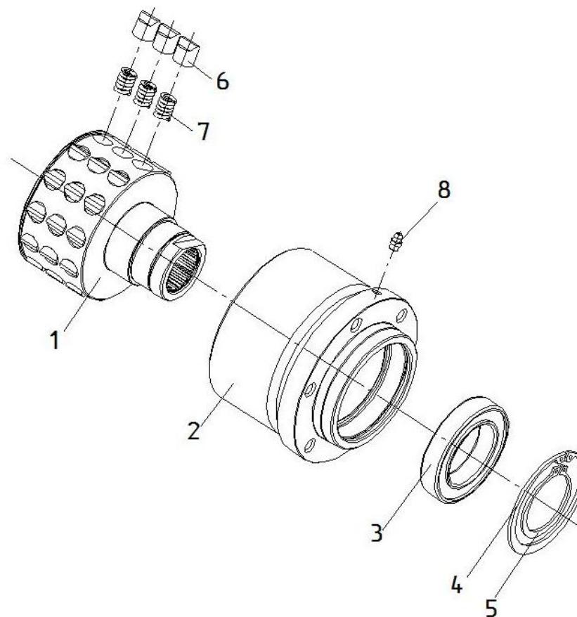
Рис. 27 Муфта предохранительная ЖК-82.00.120
