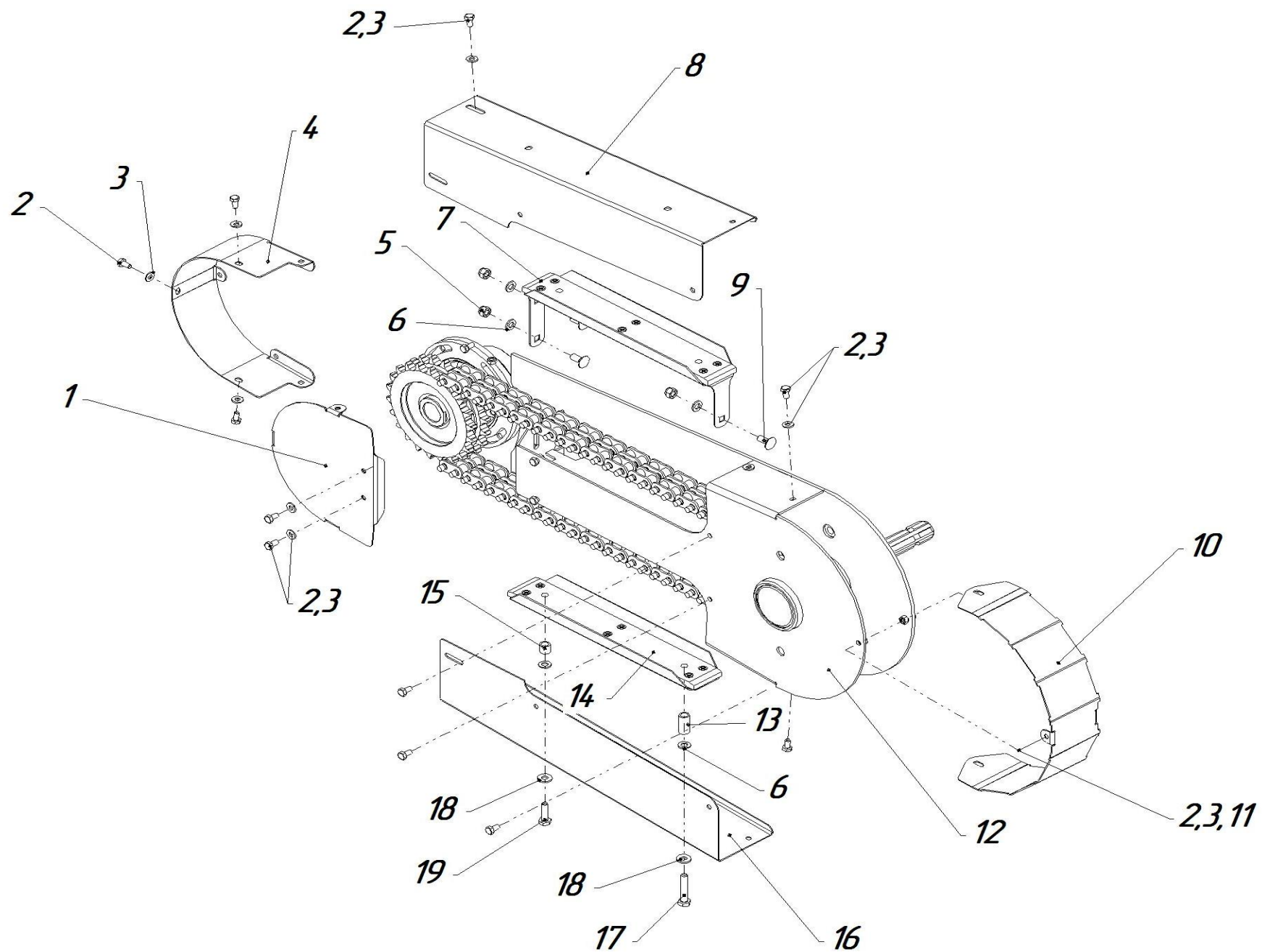
Рисунок 9 Привод ЖК- 82.03.000
