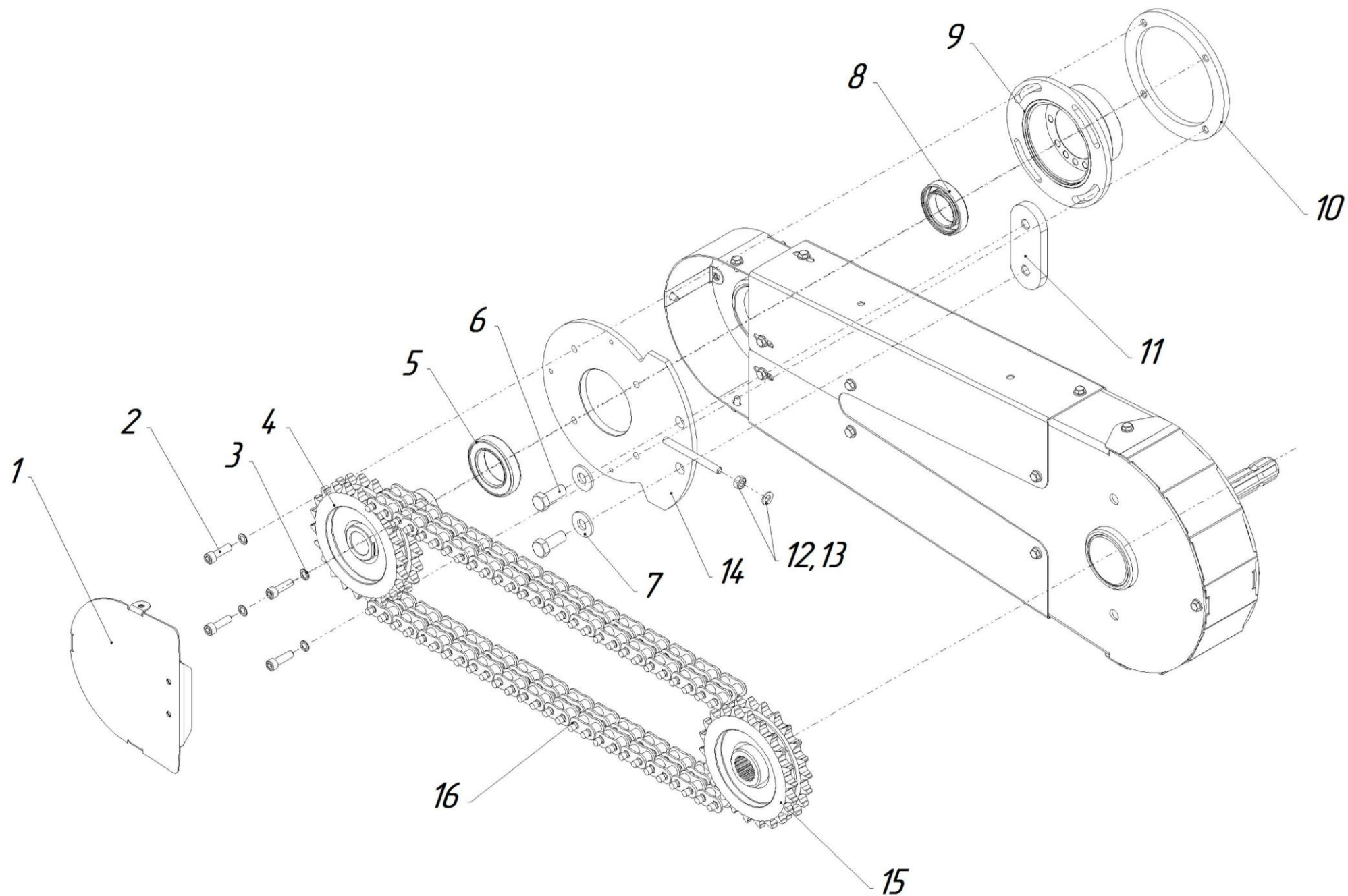
Рисунок 8 Привод ЖК- 82.03.000 (привод редукторов)
