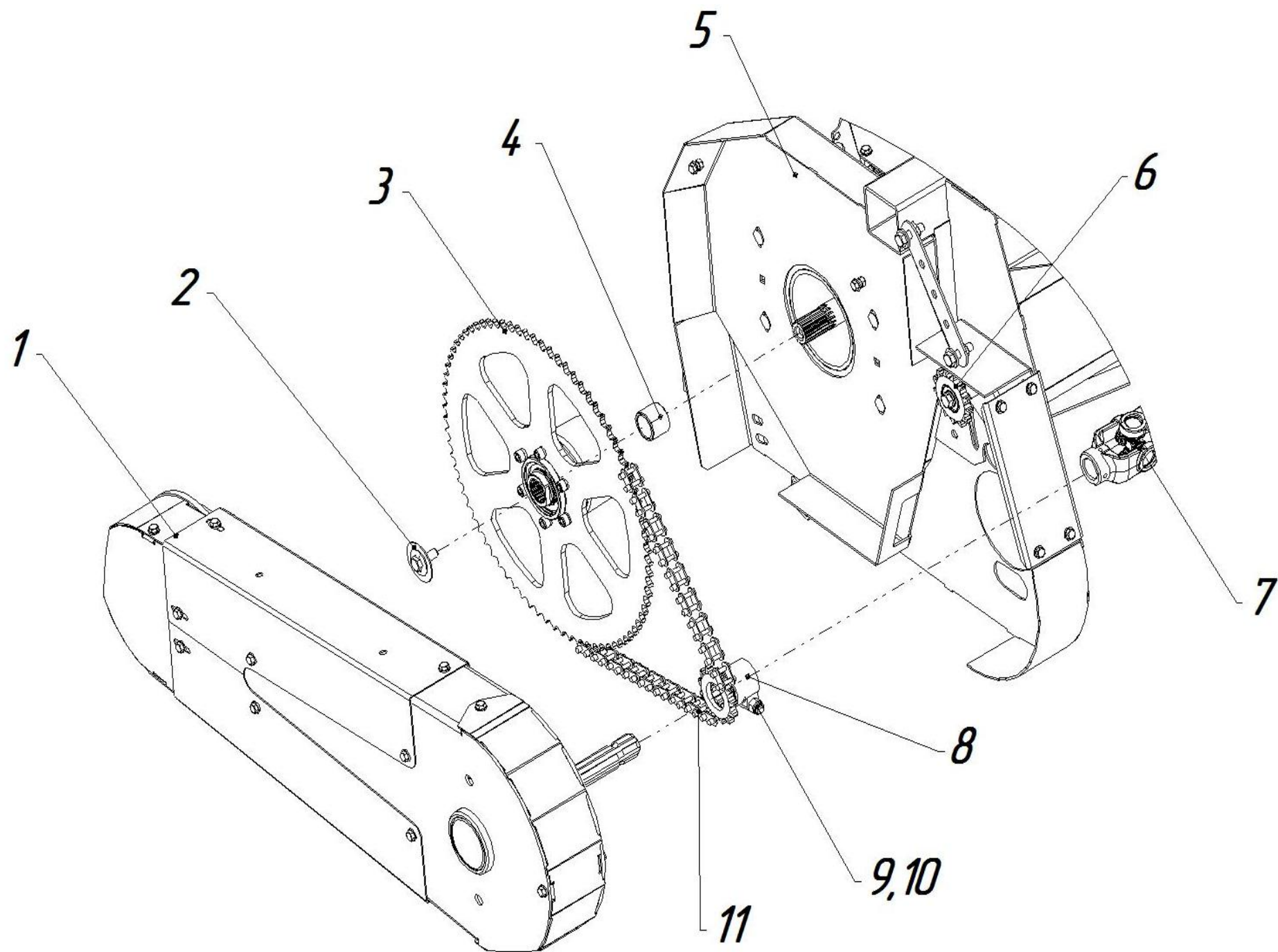
Рисунок 3 Привод шнека ЖК-82.06.000
