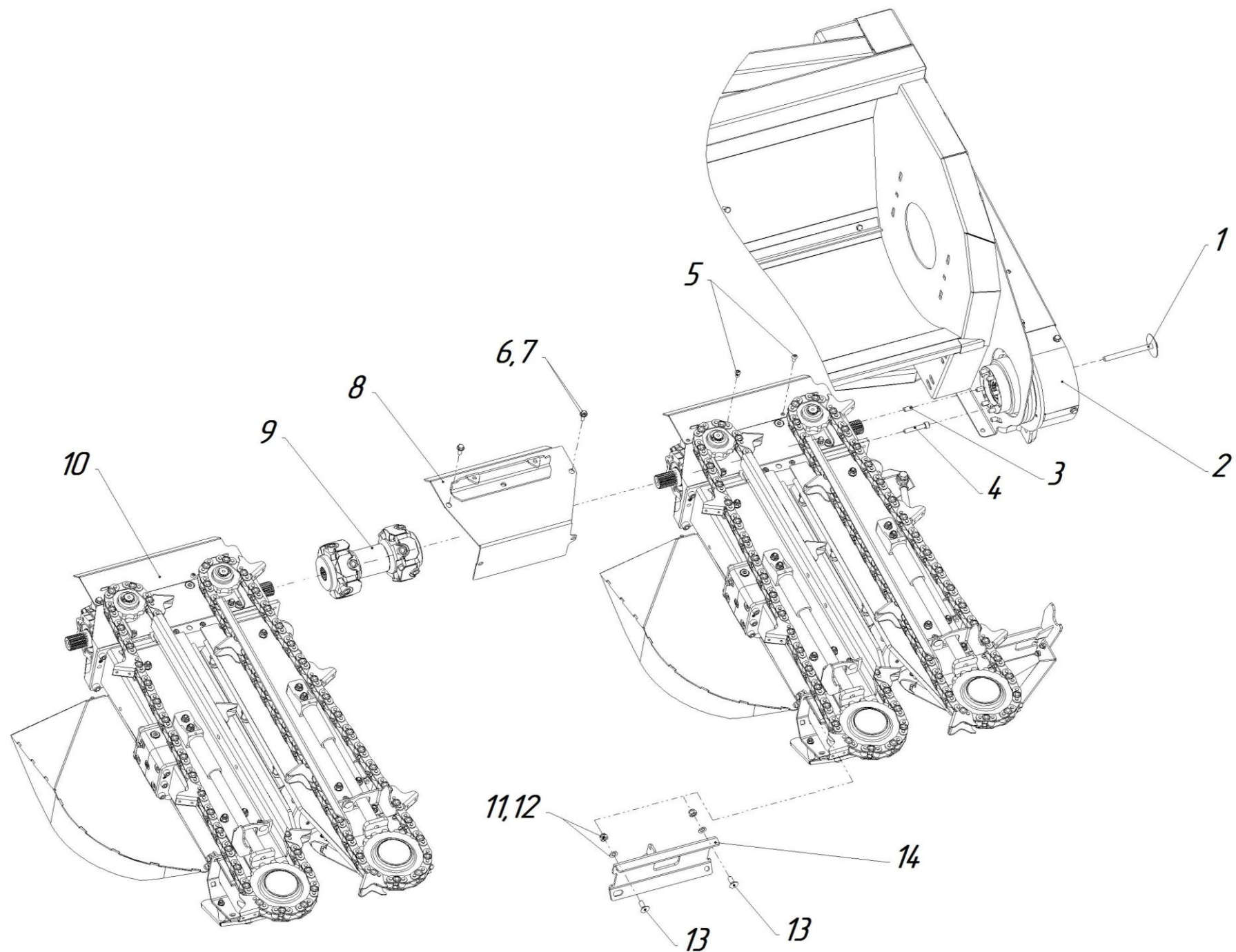
Рисунок 5 Соединение блоков режущих ЖК-82.00.000
