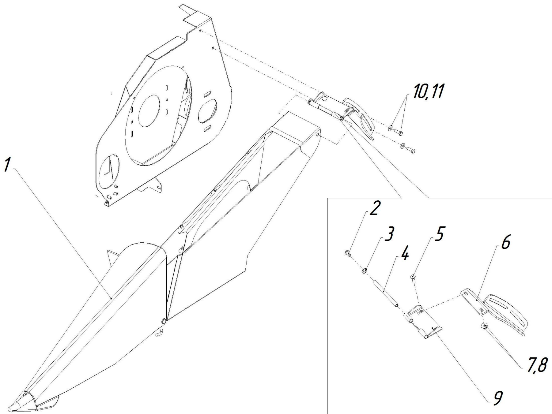
Рисунок 30 Установка делителя бокового ЖК-82.09.000(-01)
