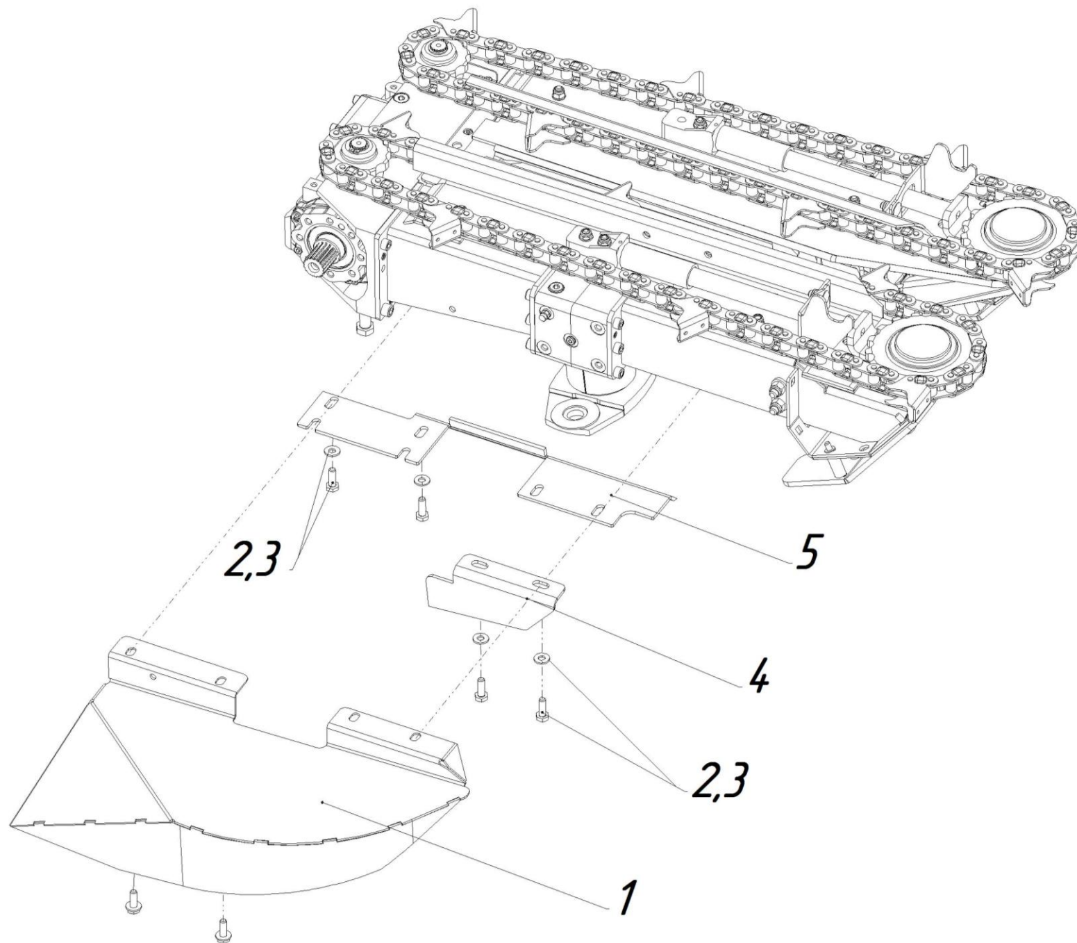
Рисунок 18 Блок режущий ЖК- 82.05.000 (Установка кожуха ЖК-82.05.800)
