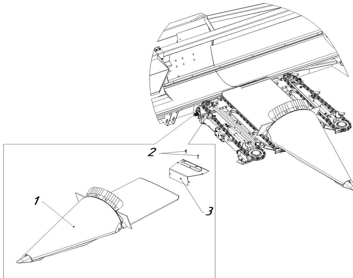
Рисунок 28 Установка делителя ЖК-80.08.000-01
