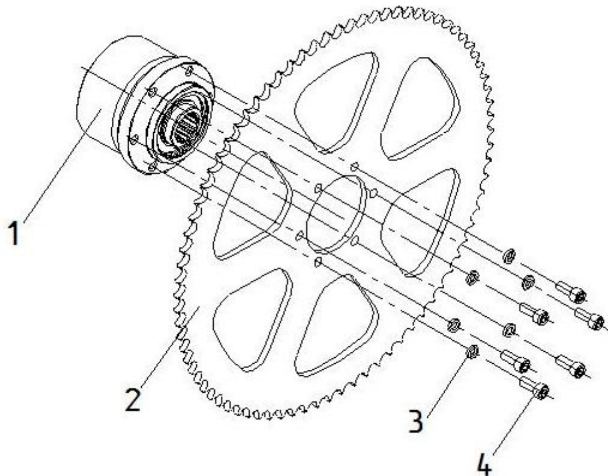
Рис. 26 Звездочка предохранительная ЖК-82.00.100
