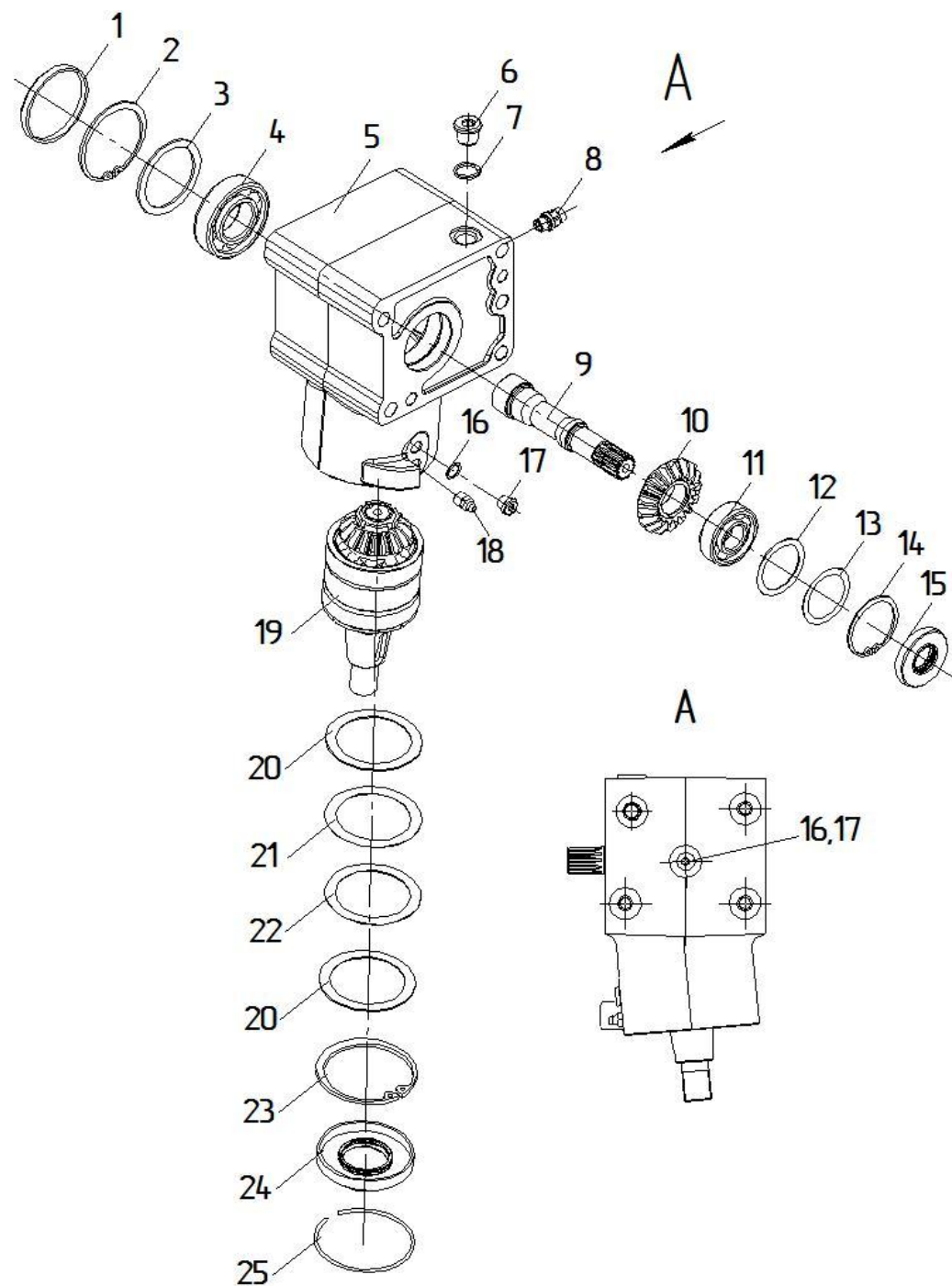
Рис. 23 Редуктор ЖК-82.04.500
