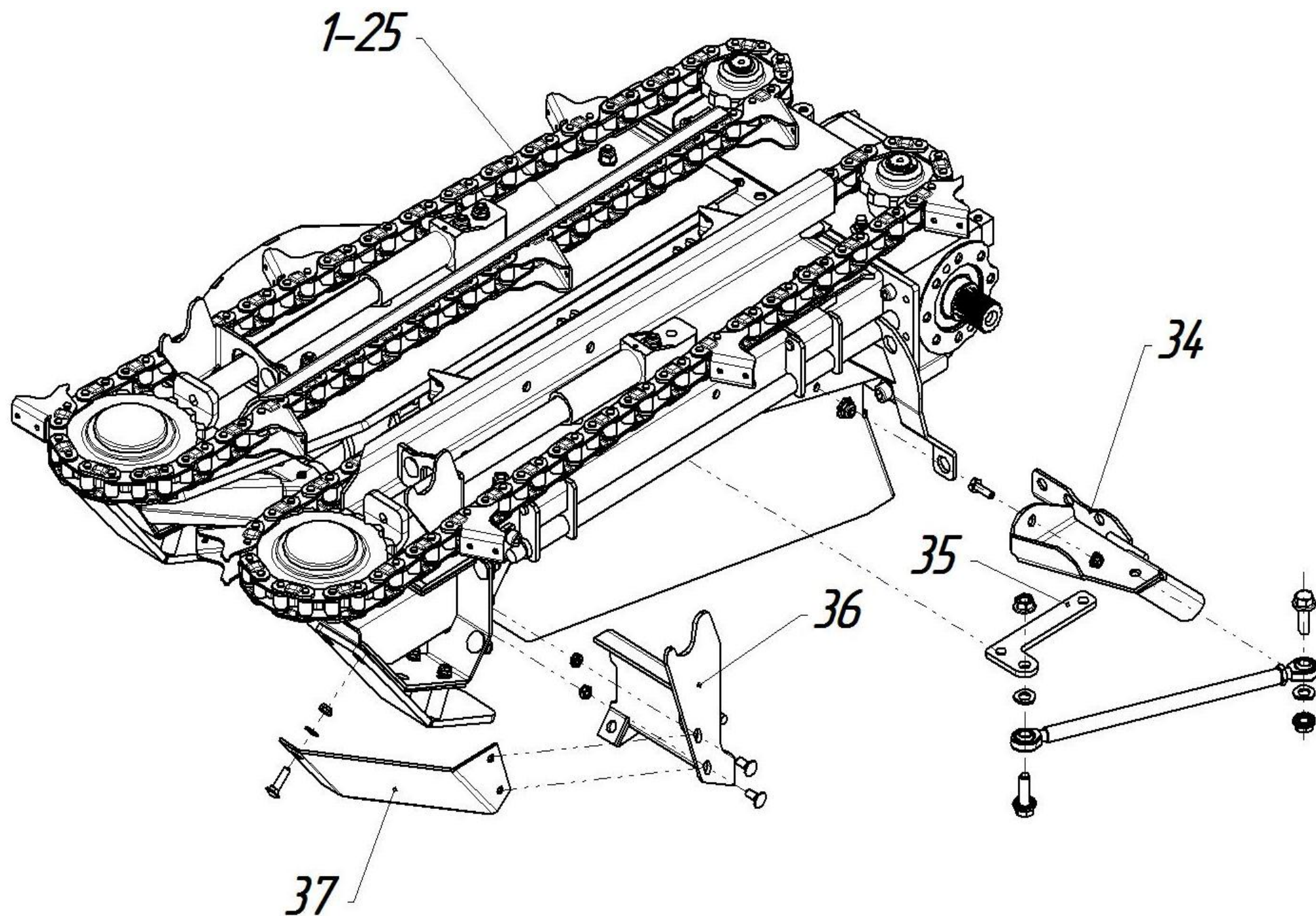
Рисунок 12 Блок режущий ЖК- 82.05.000 (-02)
