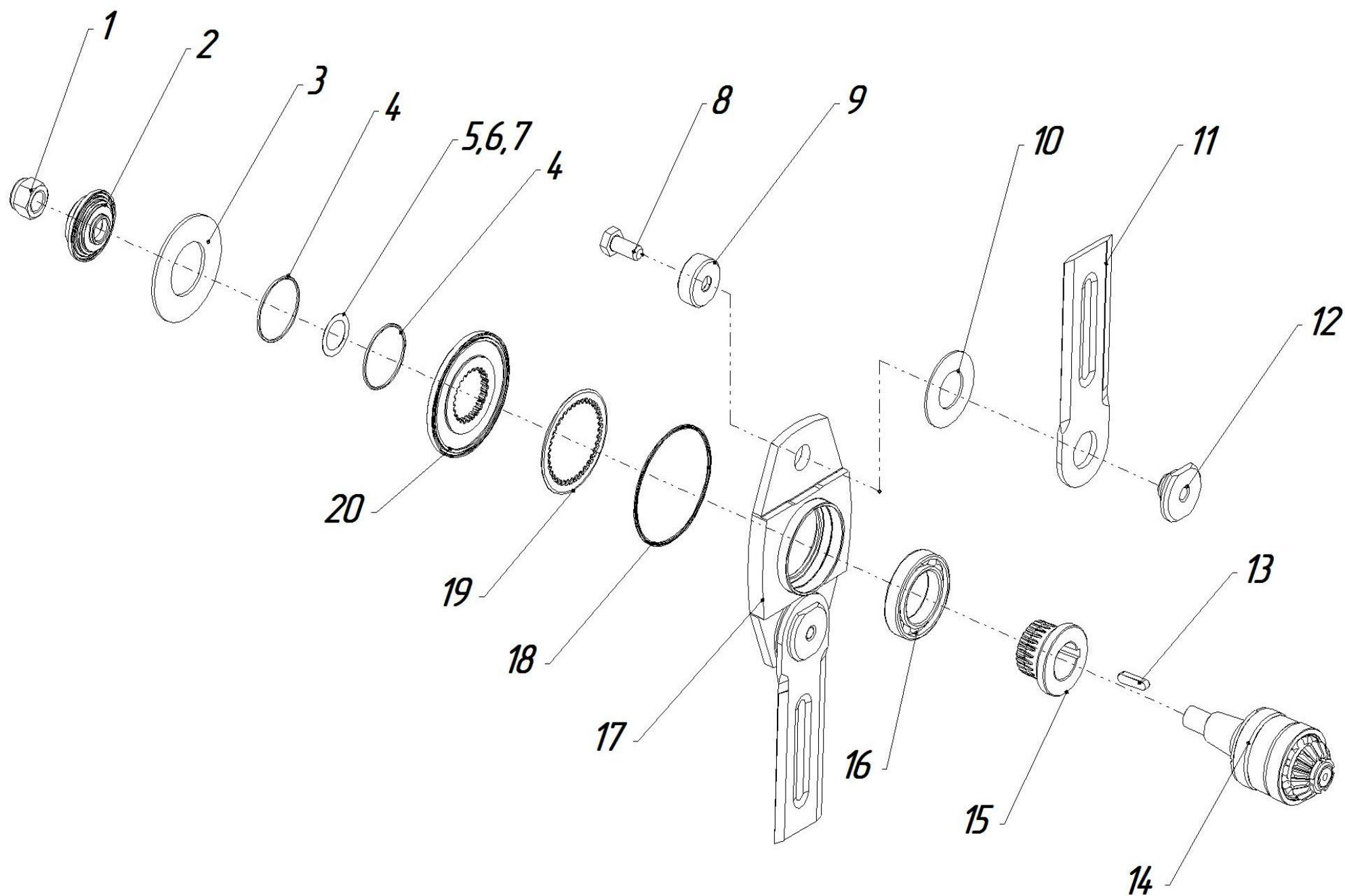
Рисунок 17 Редуктор ЖК- 82.05.000
