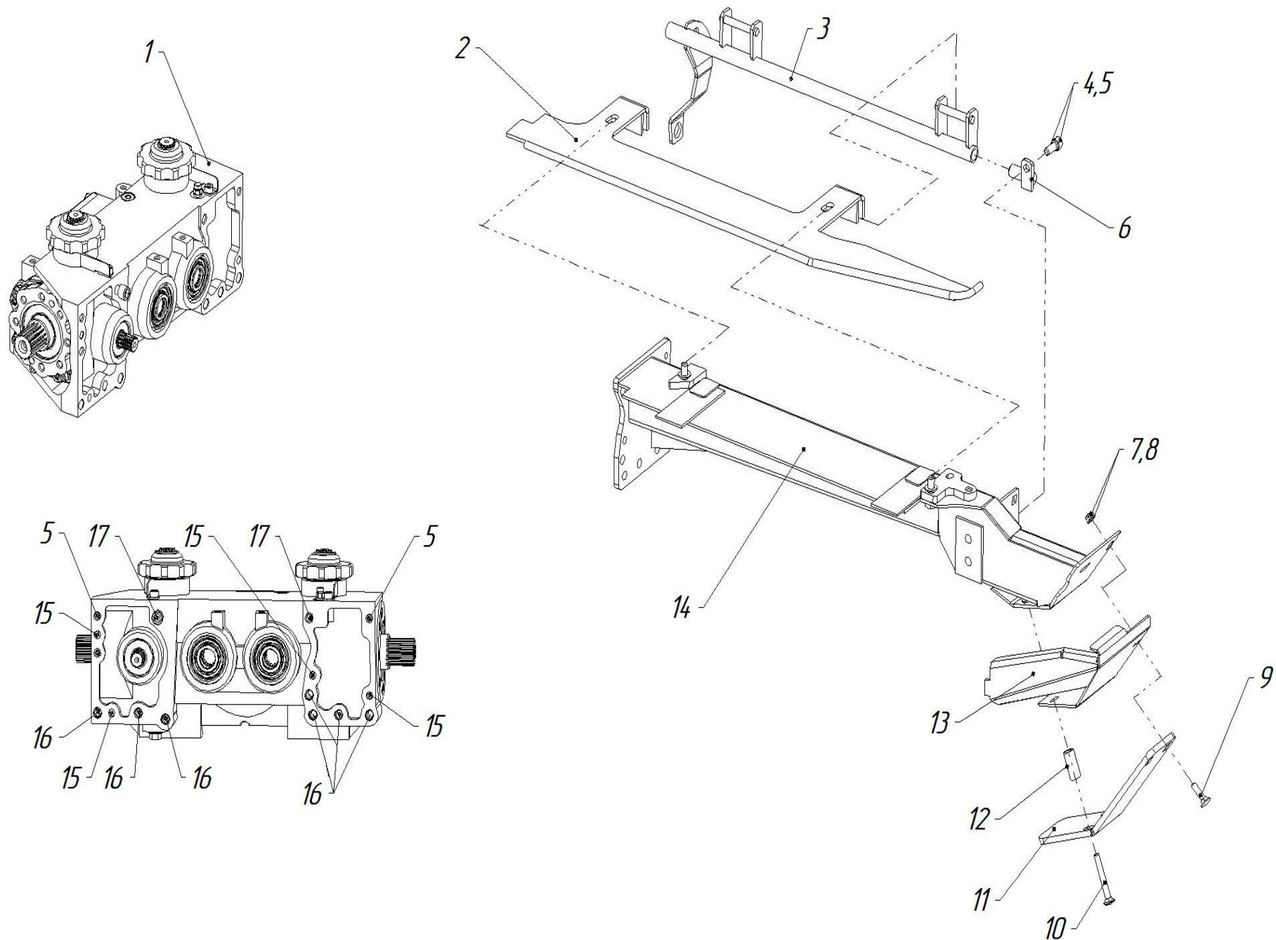
Рисунок 13 Блок режущий ЖК- 82.05.000 (Установка редуктора ЖК-82.04.000)
