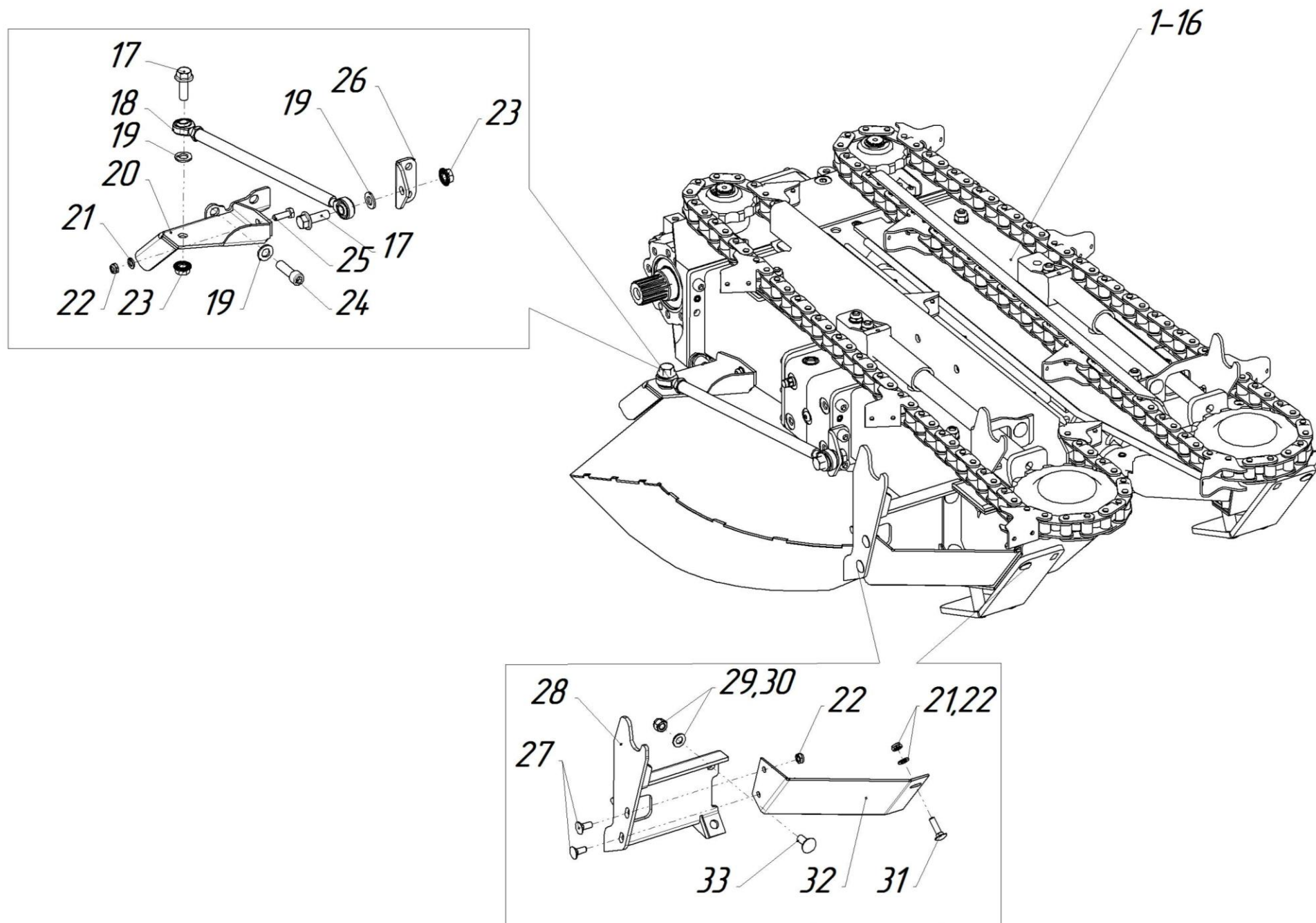
Рисунок 11 Блок режущий ЖК-82.05.000 (- 01)
