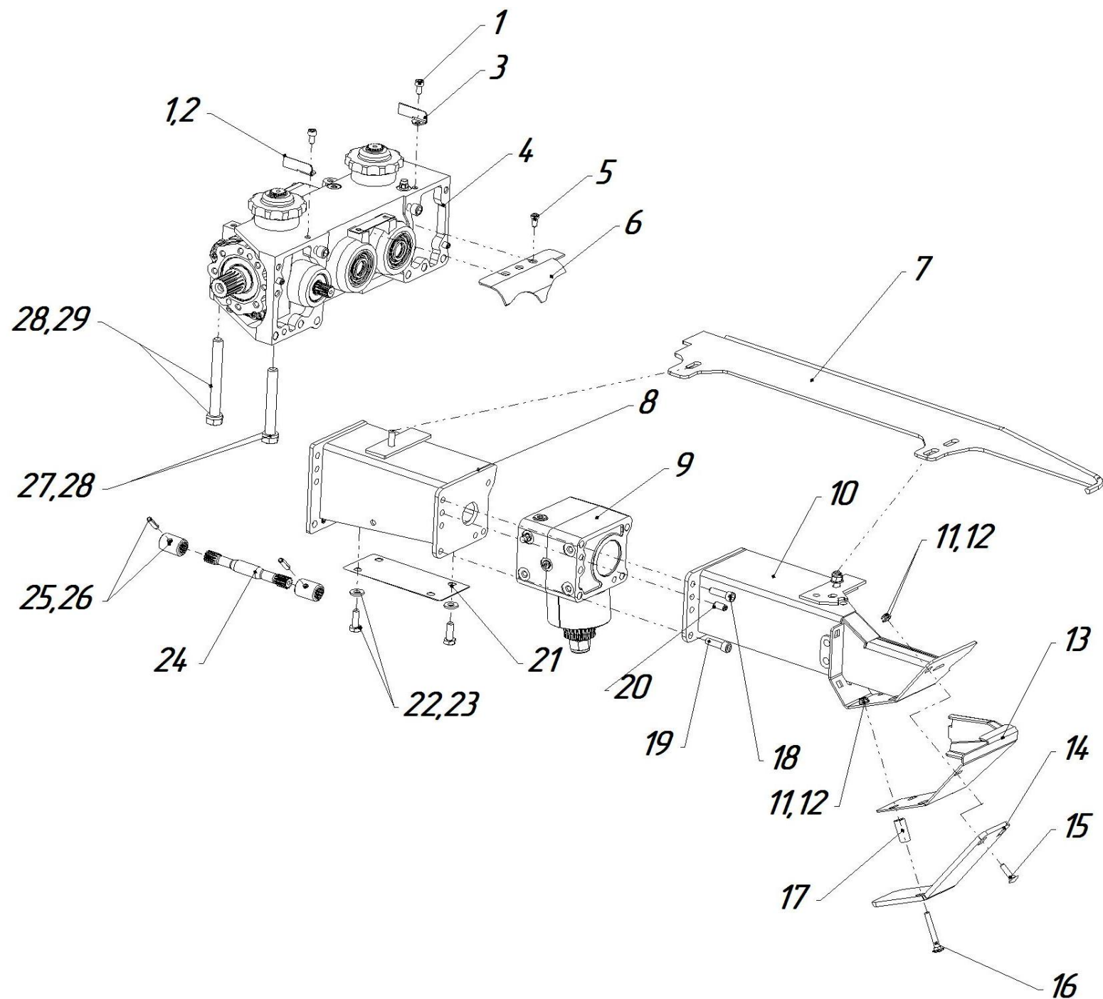
Рисунок 14 Блок режущий ЖК- 82.05.000 (установка редуктора измельчителя ЖК-82.04.500)
