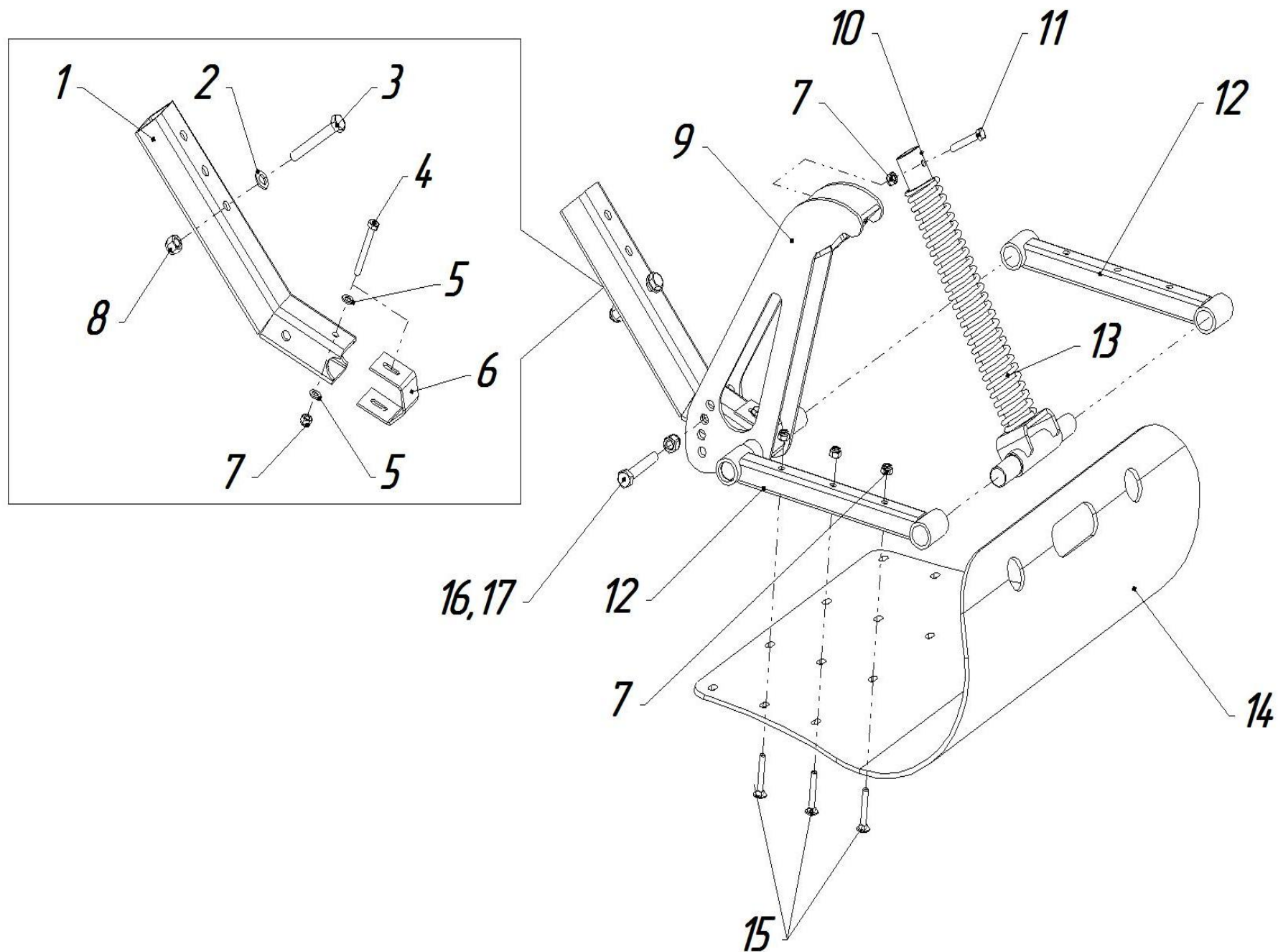
Рисунок 32 Отбойник ЖК-82.15.000
