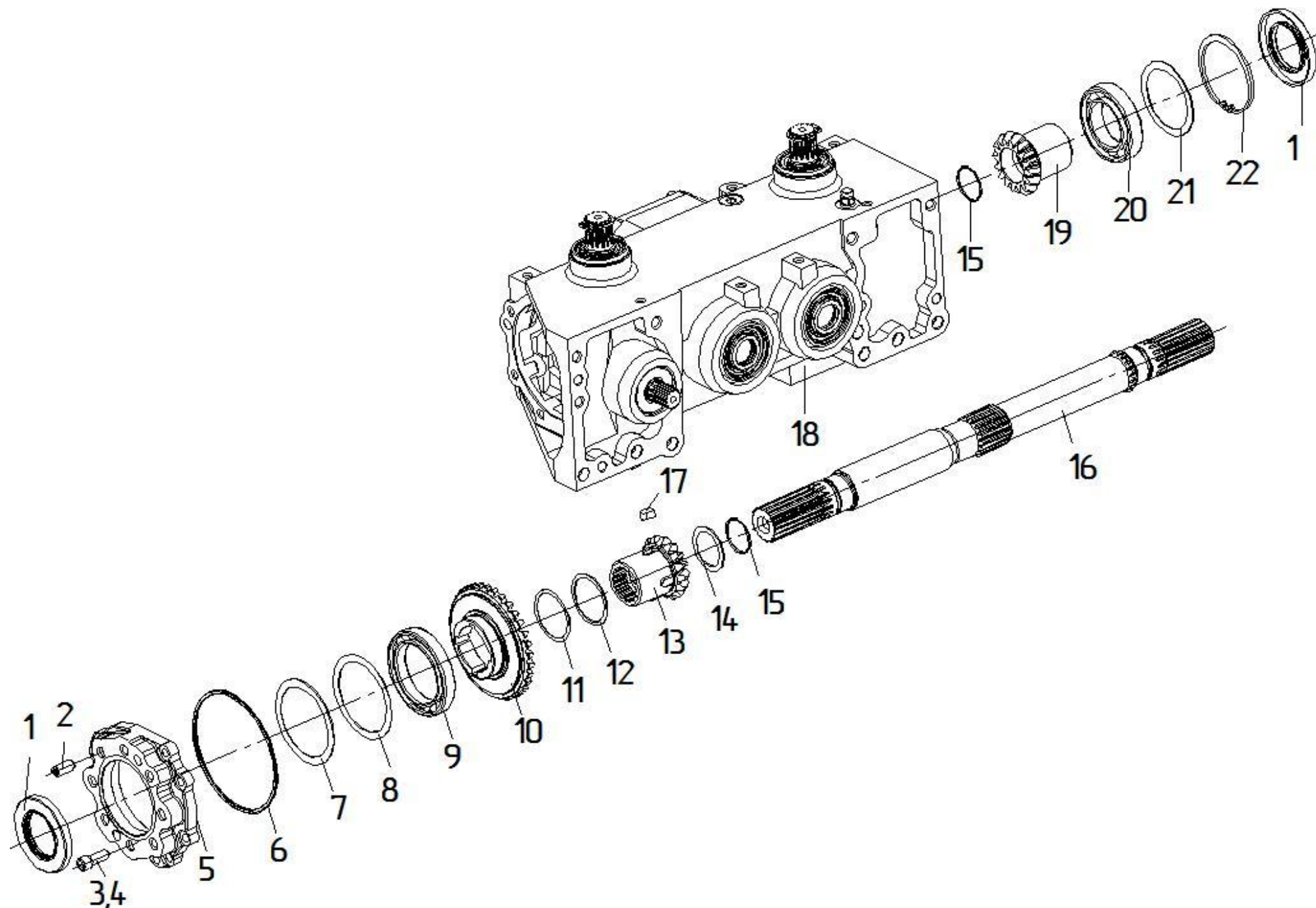
Рис. 21 Редуктор ЖК-82.04.000 (вал горизонтальный продольный)
