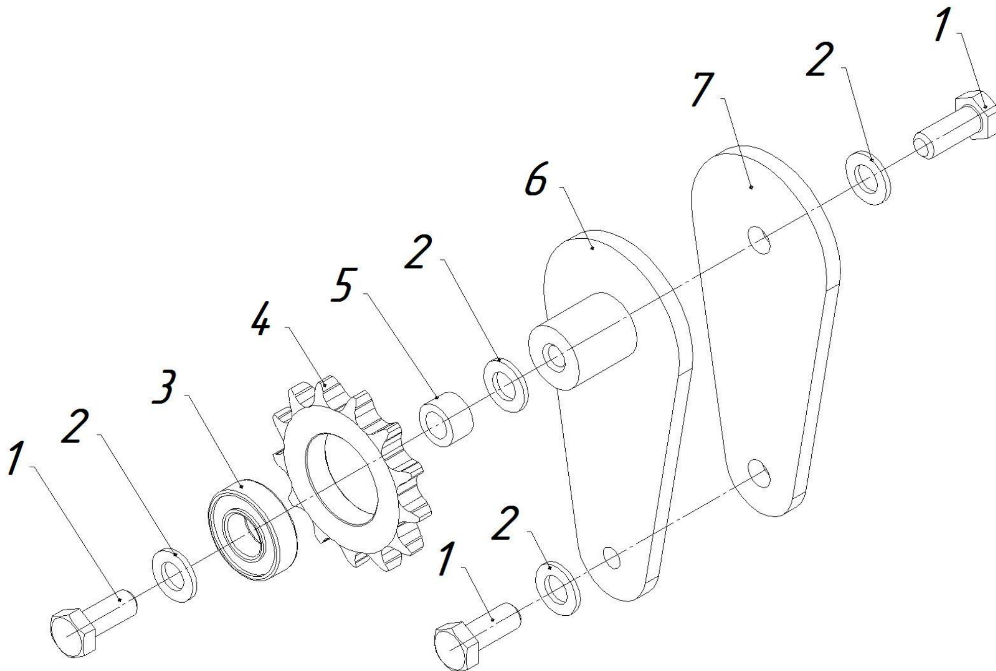
Рисунок 4 Звездочка натяжная ЖК-82.01.300
