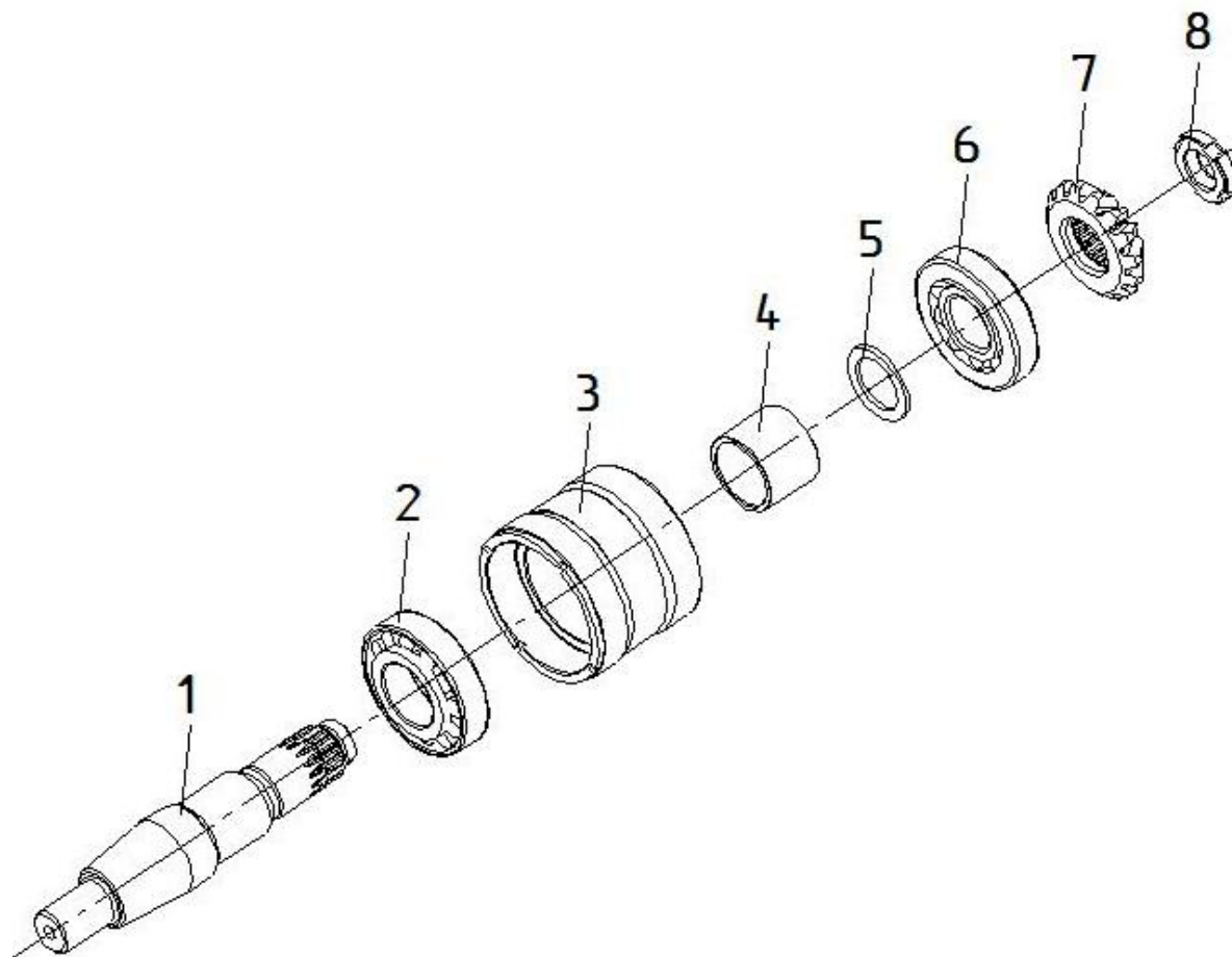
Рис. 24 Блок ЖК-82.04.600-01
