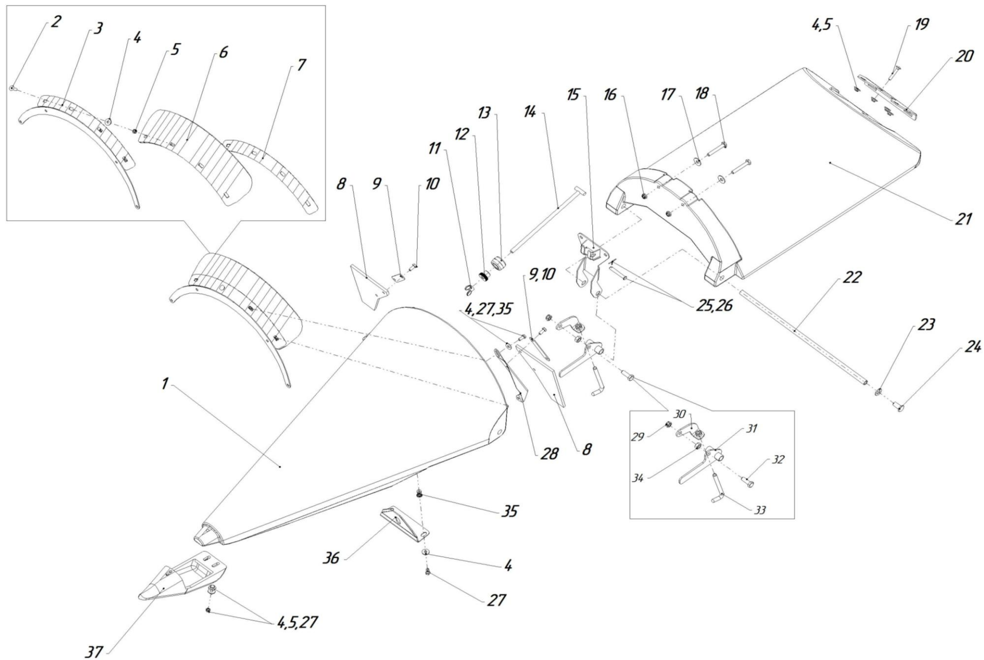
Рисунок 29 Делитель ЖК- 80.08.000(-01)
