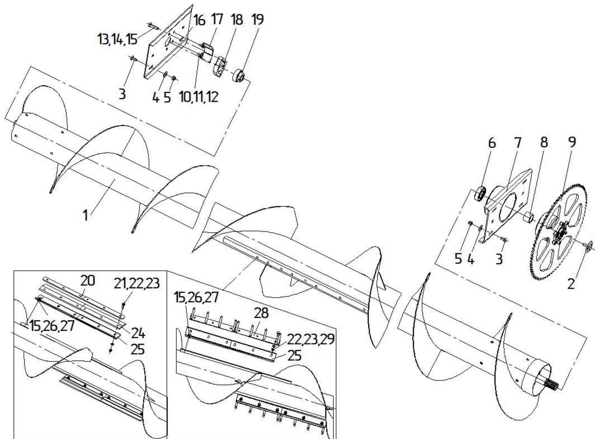
Рис. 25 Шнек ЖК-82.06.000
