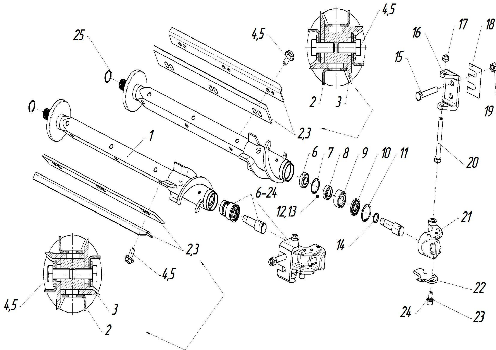
Рисунок 15 Установка вала ЖК-82.05.500-02(-03)
