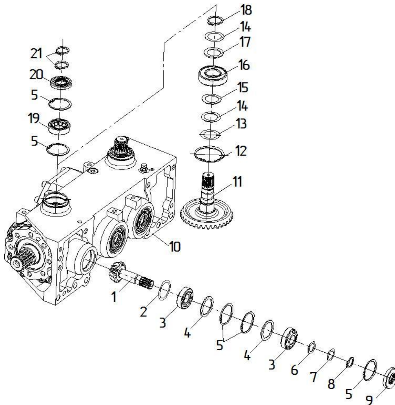
Рис. 22 Редуктор ЖК-82.04.000 (вал горизонтальный поперечный и вертикальный)
