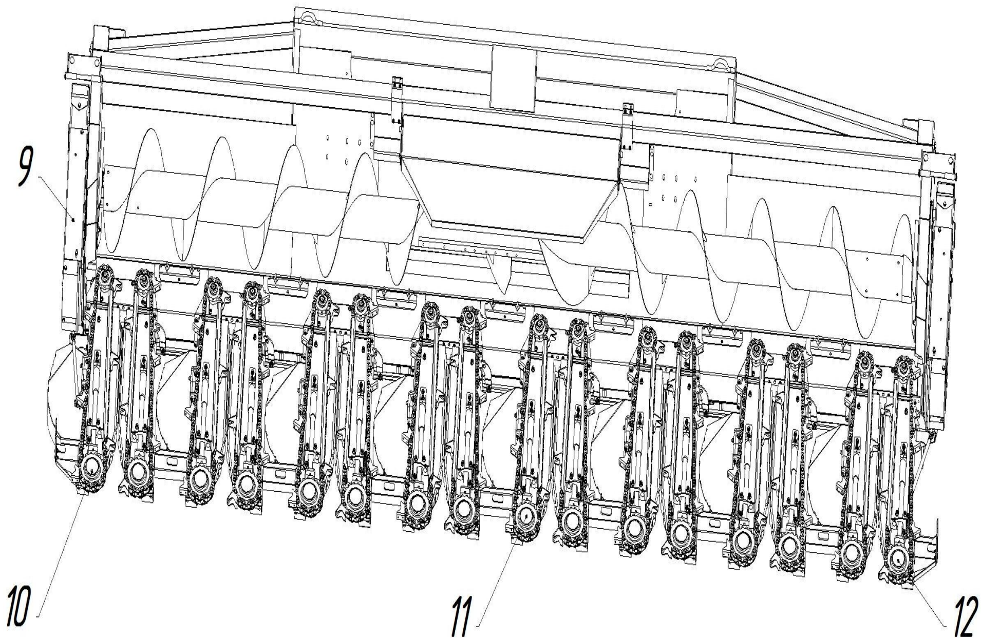
Рисунок 2 Общий вид жатки ЖК- 82.00.000
