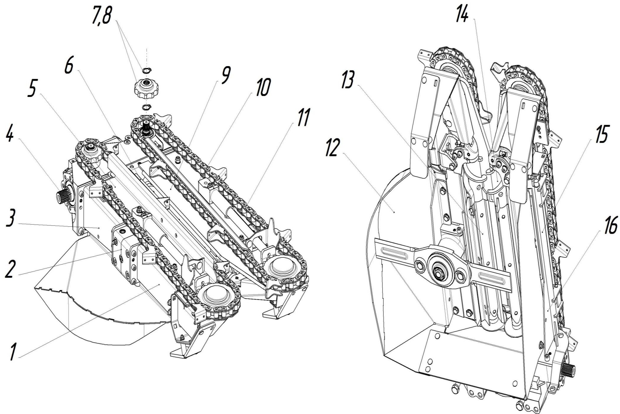
Рисунок 10 Блок режущий ЖК-82.05.000
