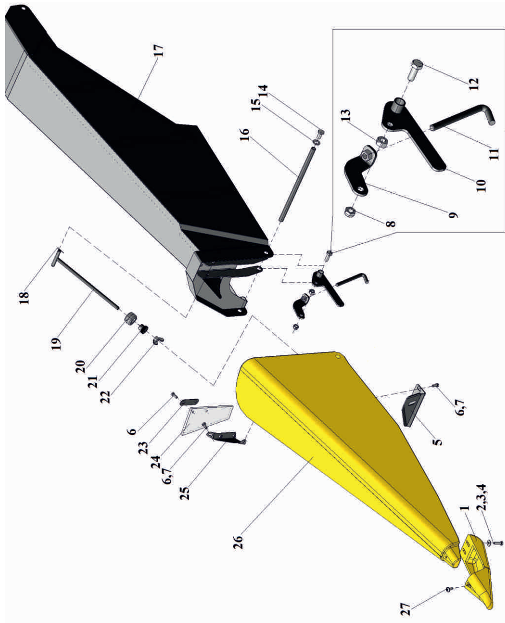
Рис. 17 Делитель ЖК-80.09.000
