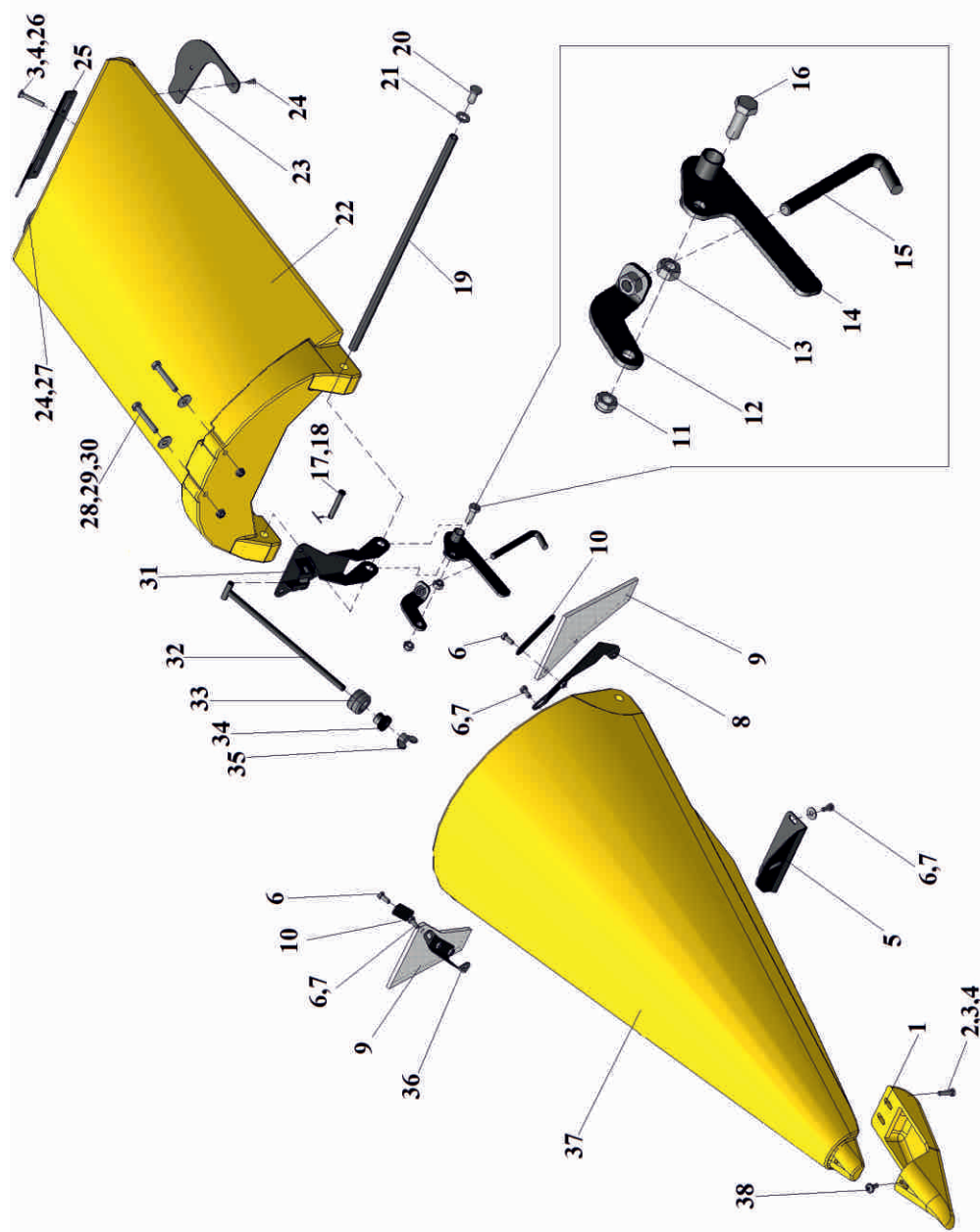
Рис. 16 Делитель ЖК-80.08.000
