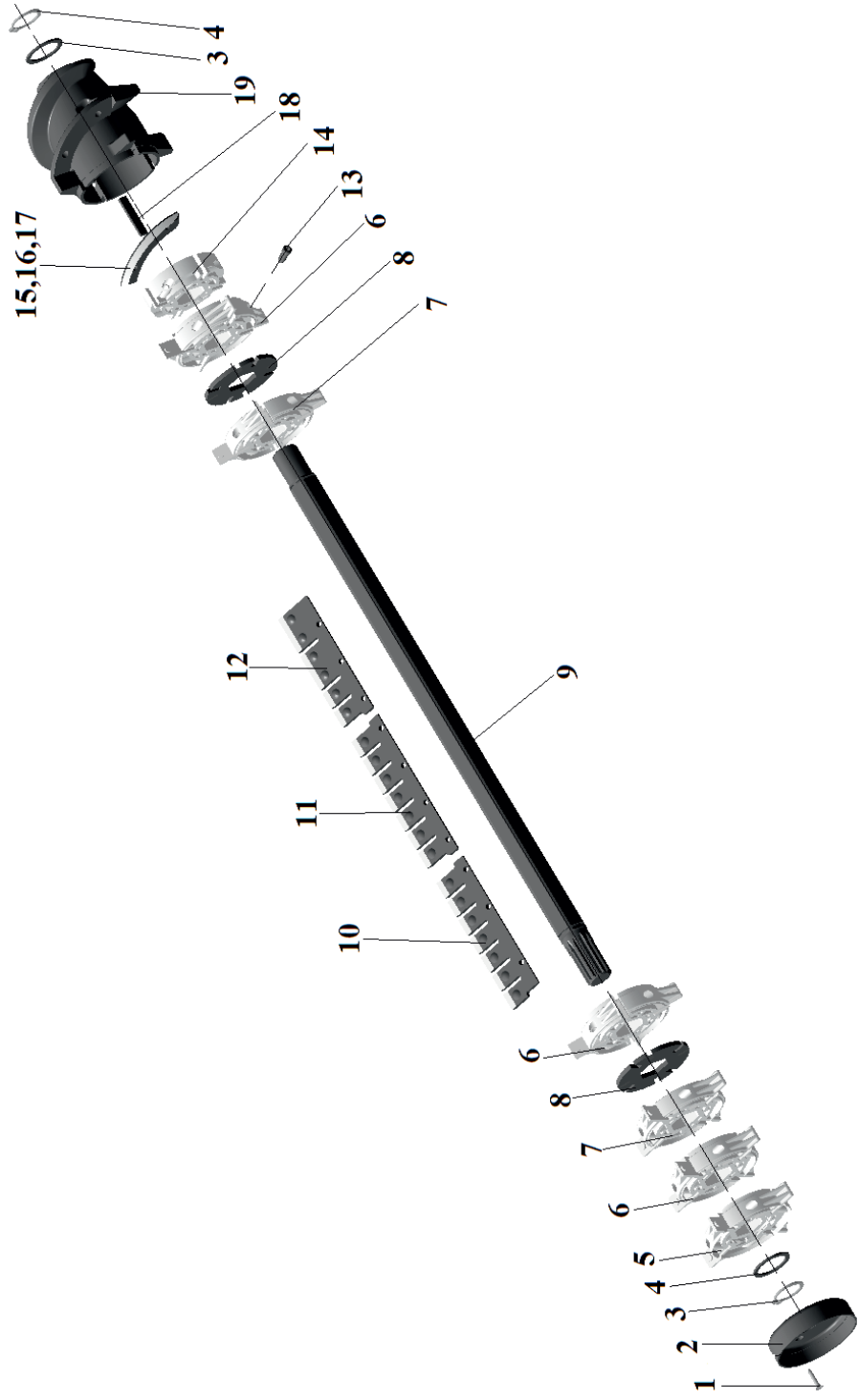
Рис. 10 Барабан ЖК-80.05.500
