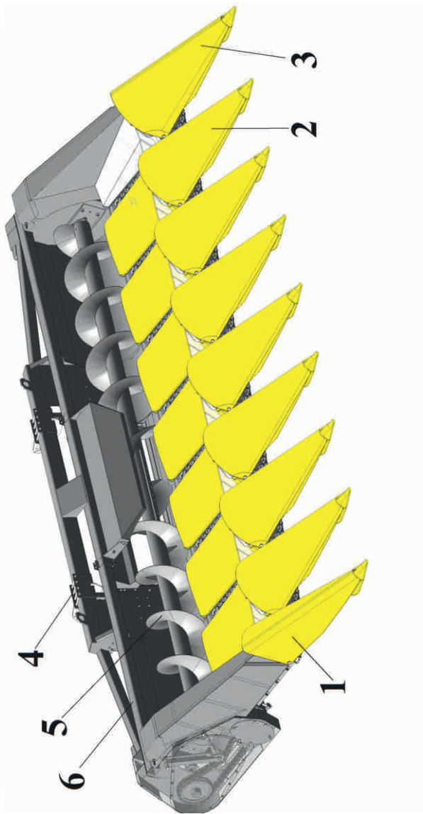
Рис. 1 Общий вид жатки 4
