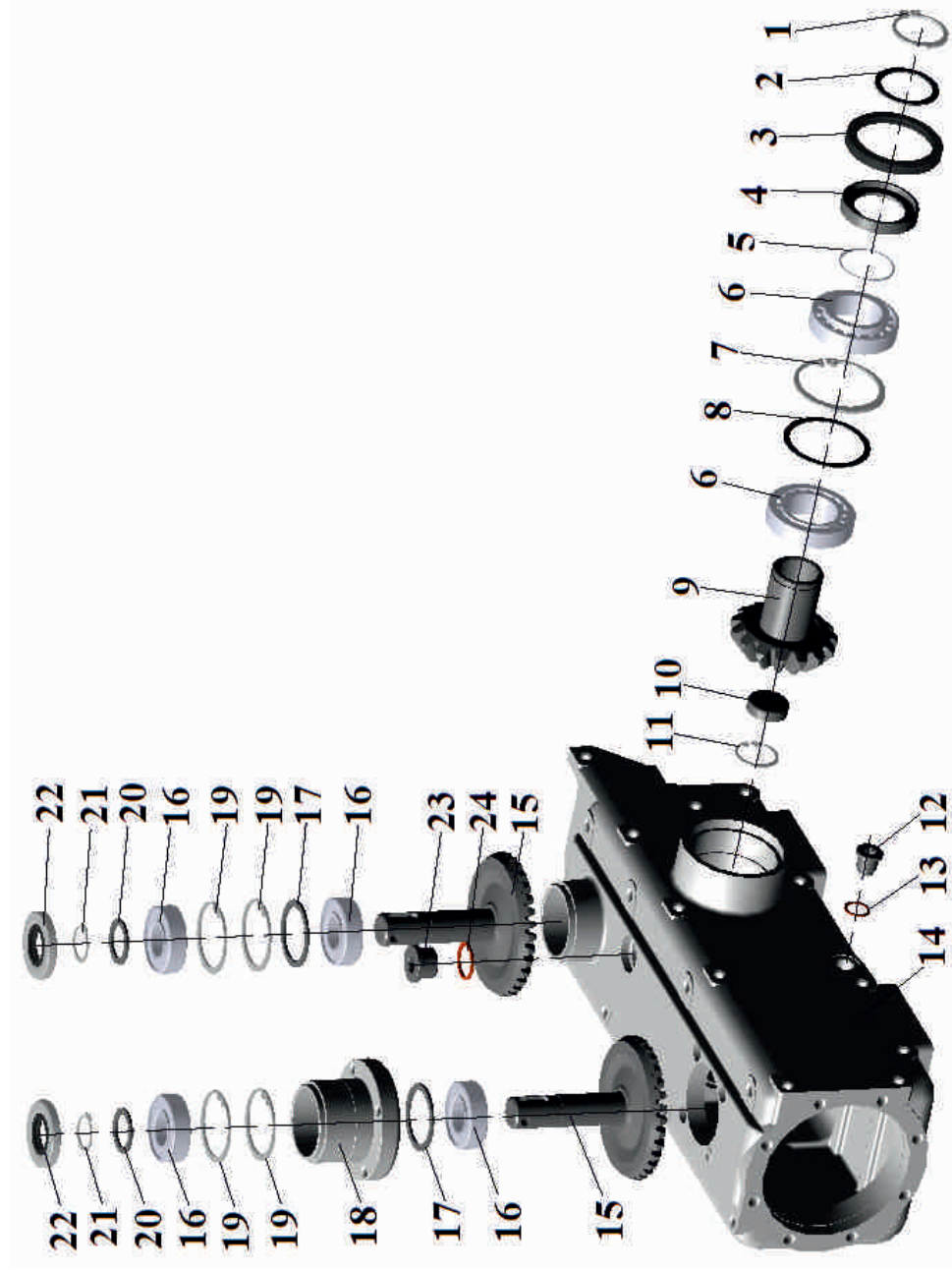
Рис. 9 Редуктор ЖК-80.04.000
