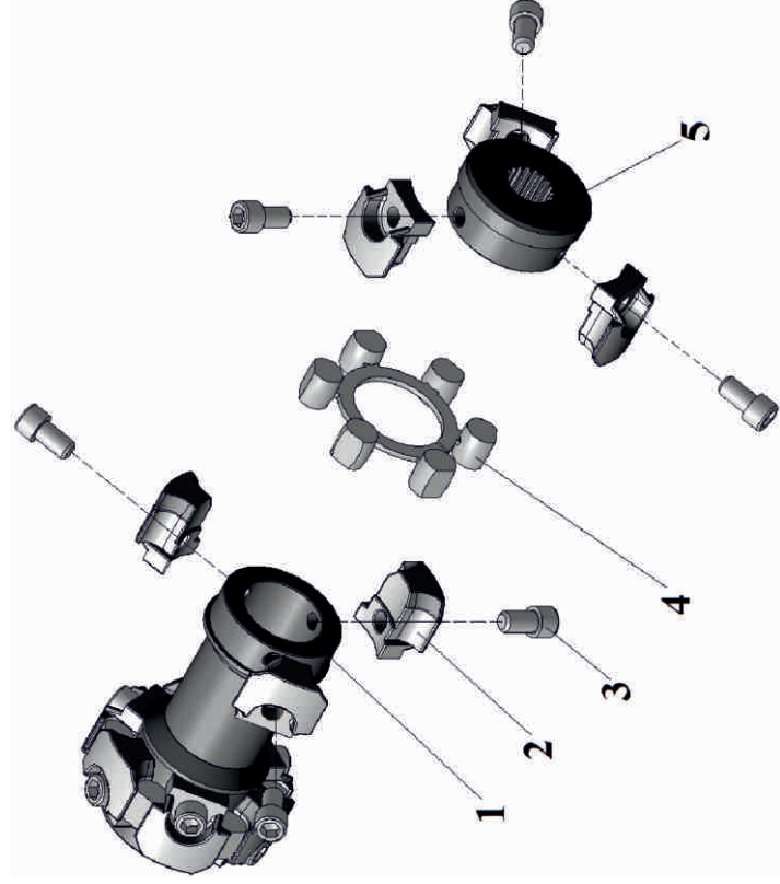
Рис. 7 Муфта соединительная ЖК-80.01.810
