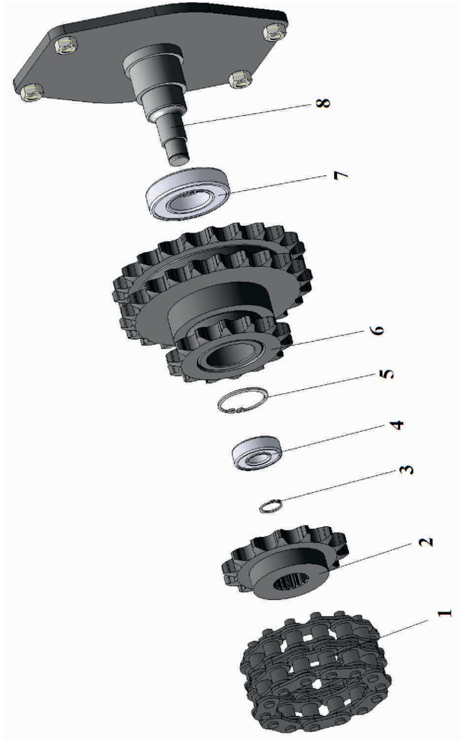
Рис. 3 Муфта цепная ЖК-80.01.820
