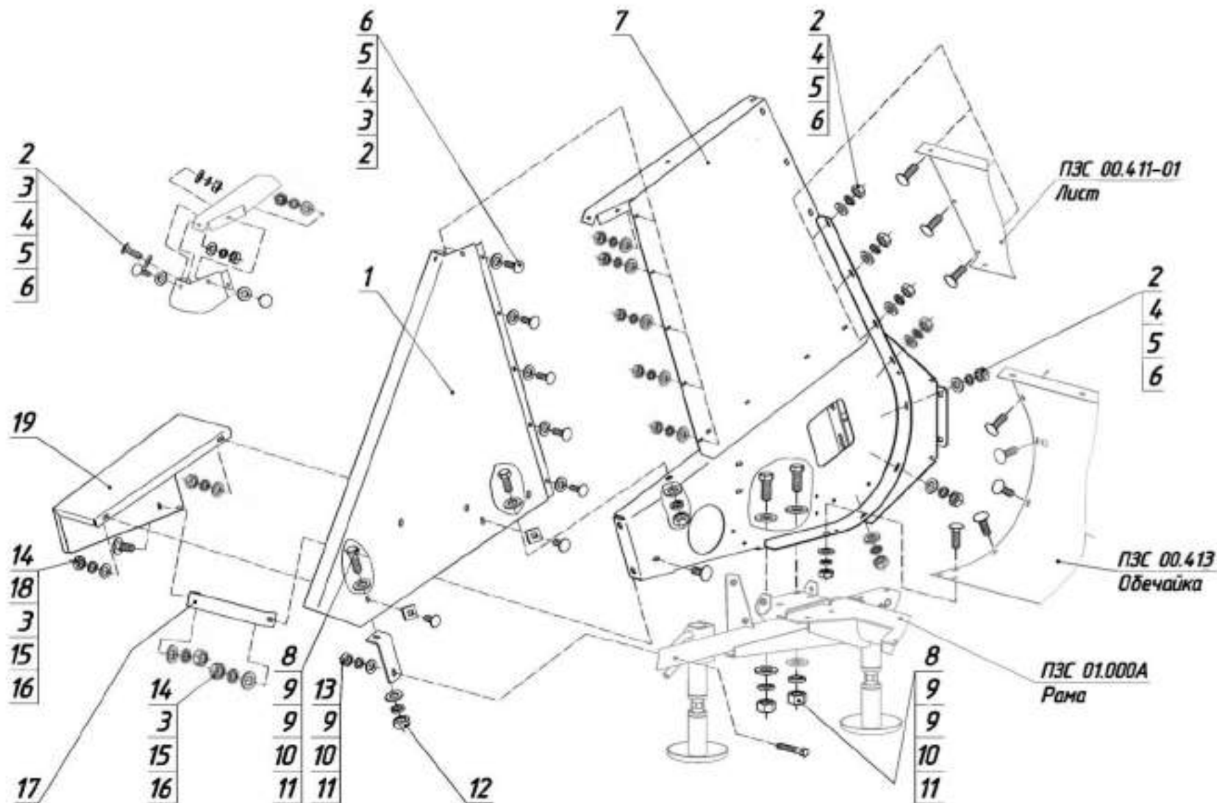
Корпус (правая сторона) (лист 1)
