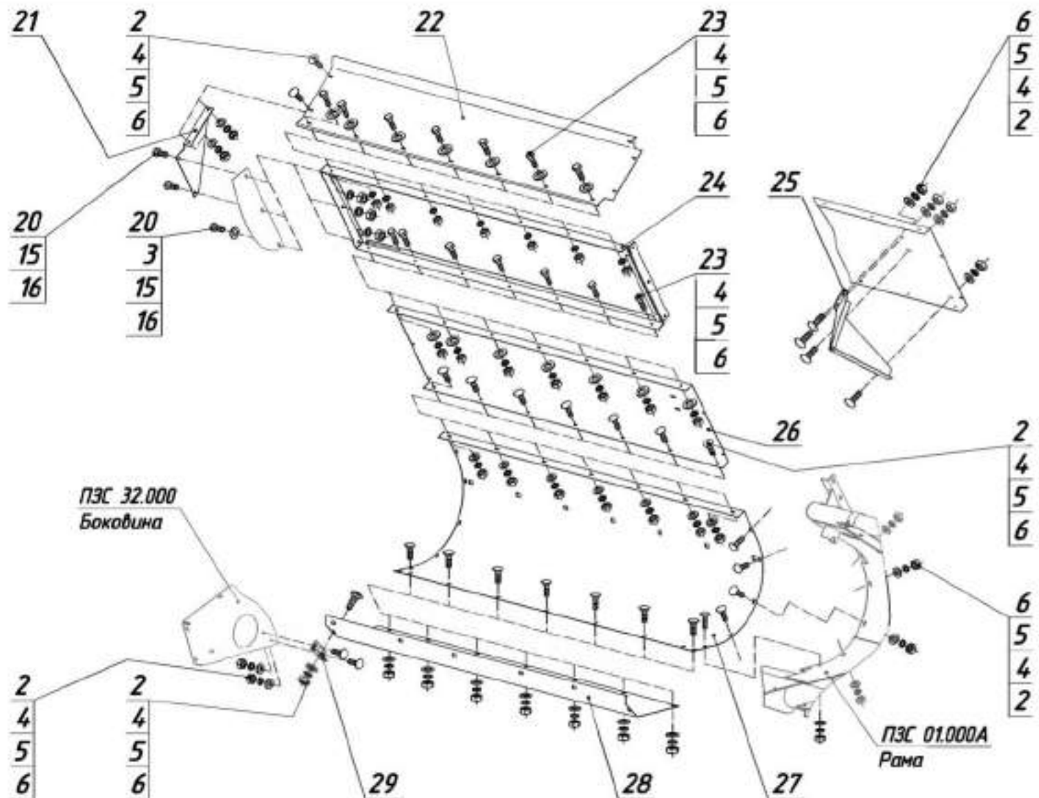
Корпус (правая сторона) (лист 2)
