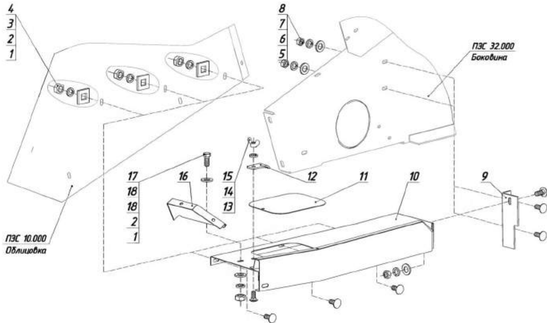
Капот ПЗС 33.000 с установленными элементами
