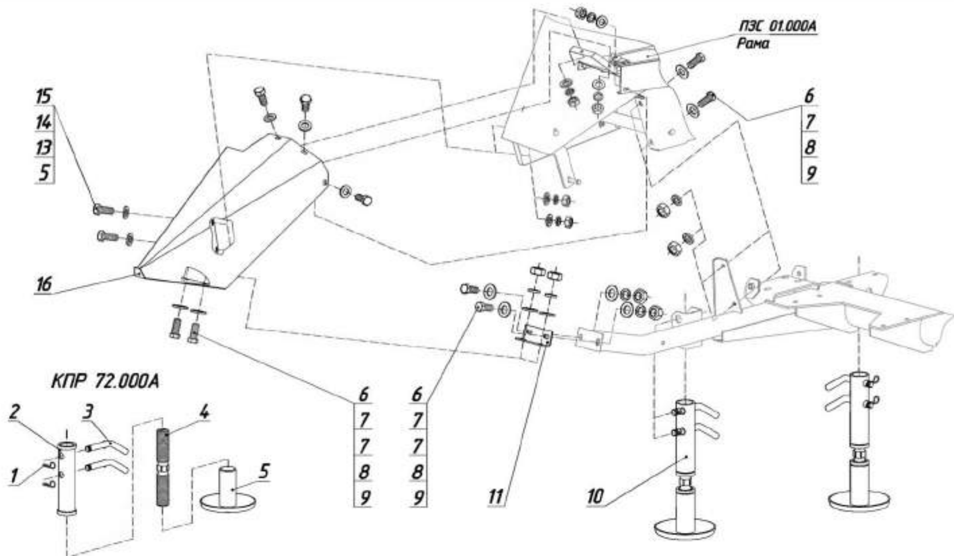
Рама ПЗС 01.000А с установленными элементами (лист 2)
