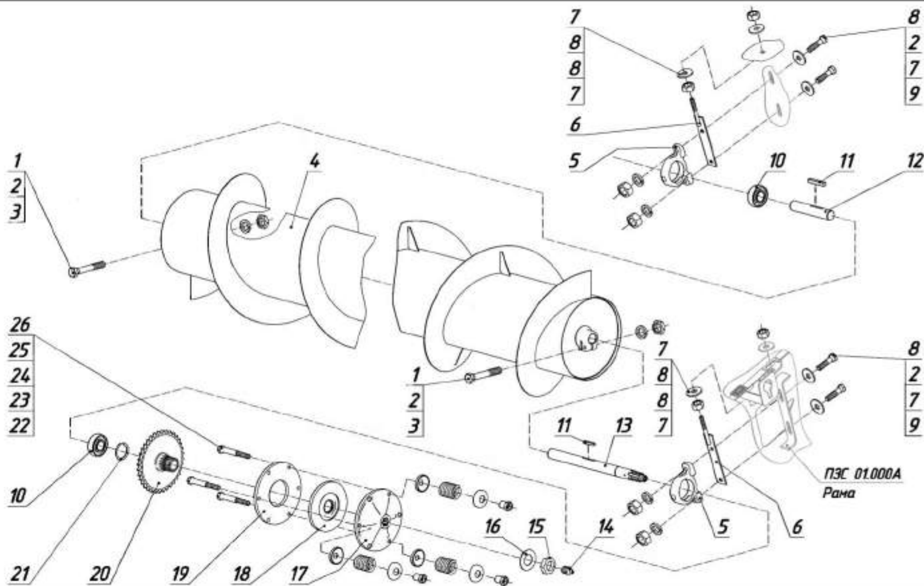
Шнек ПЭС 11.000
