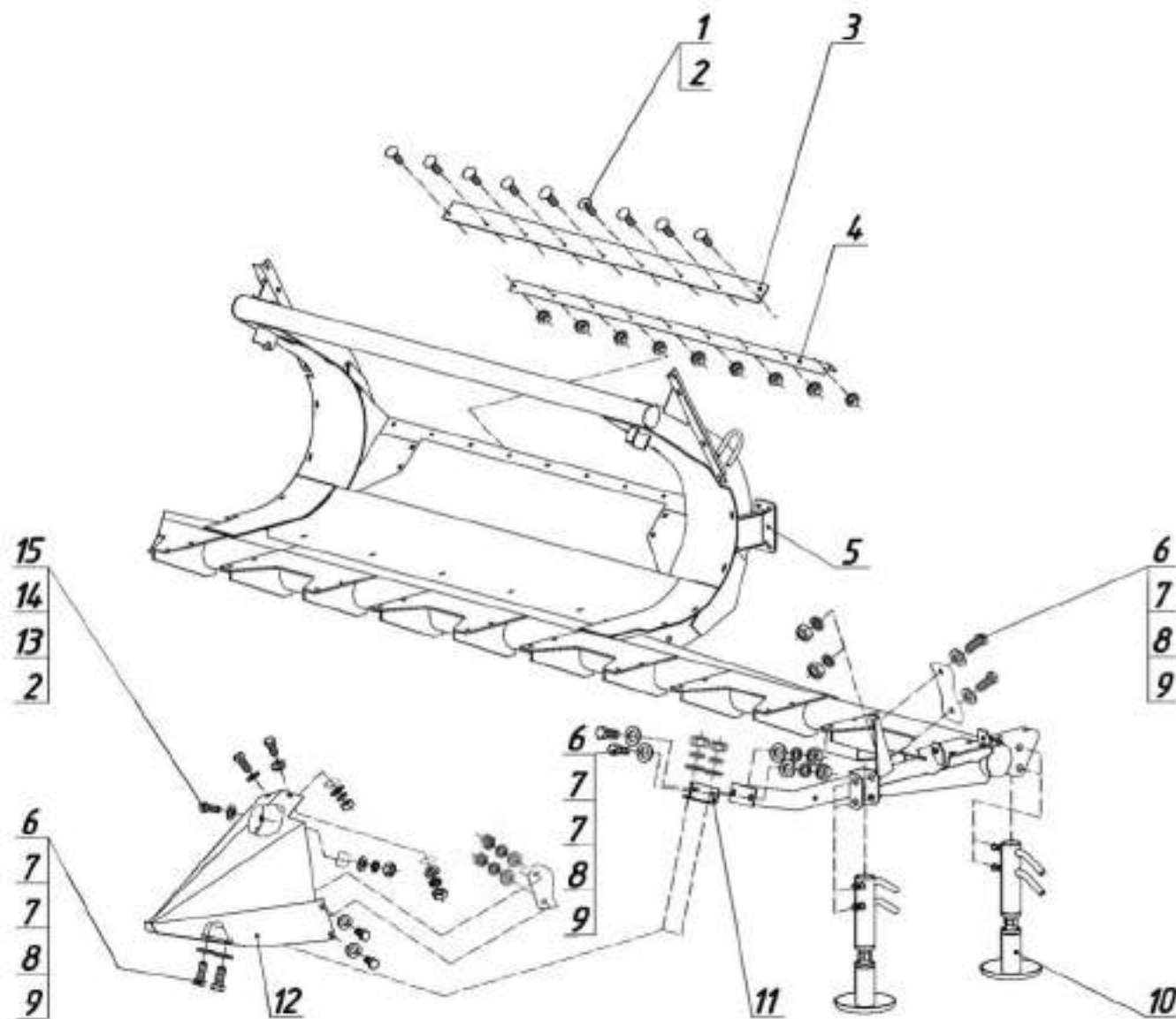
Рама ПЗС 01.000А с установленными элементами (лист 1)
