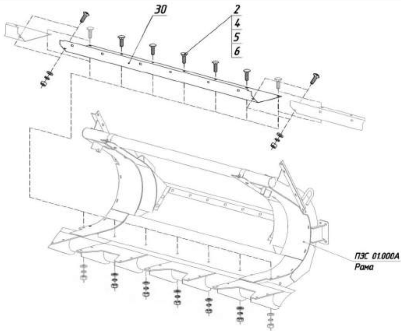
Корпус (правая сторона) (лист 3)
