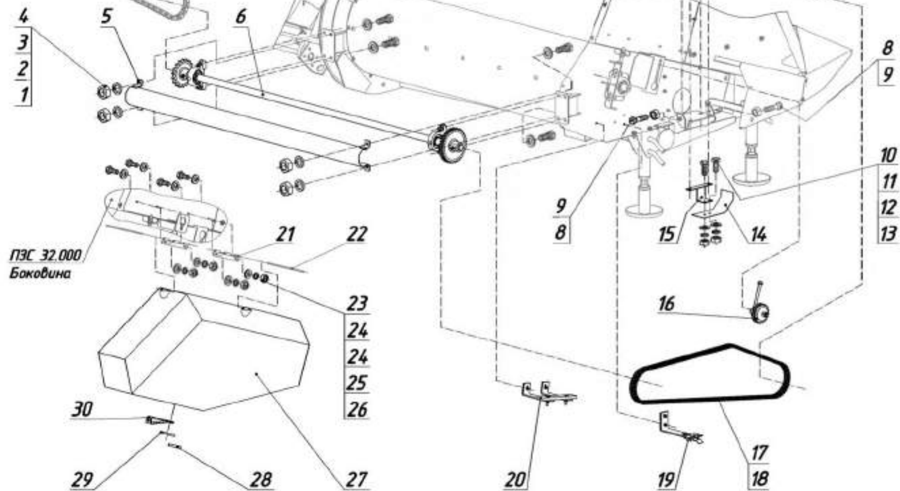
Привод (правая сторона) с ограждением ПЭС 18.000А-01
