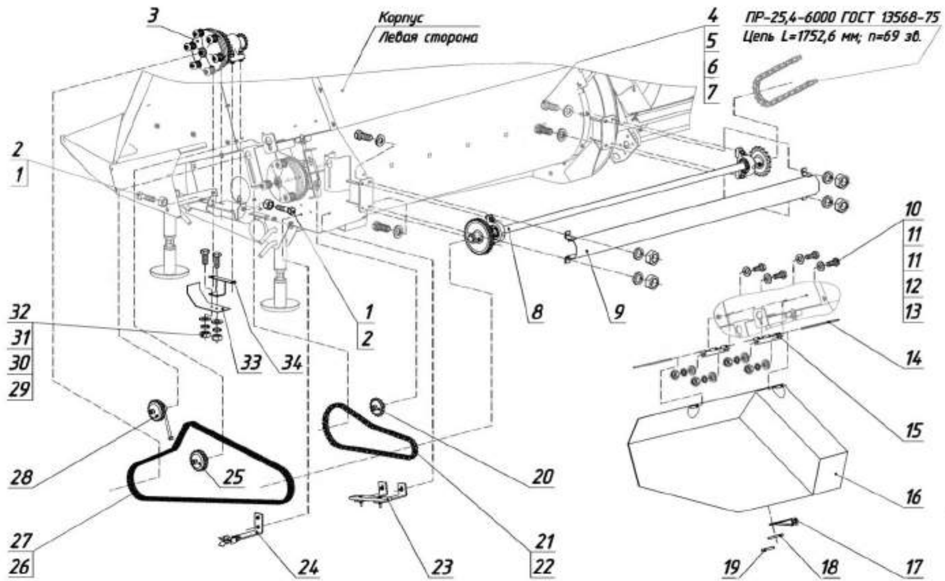
Привод (левая сторона) с ограждением ПЭС 18.000А
