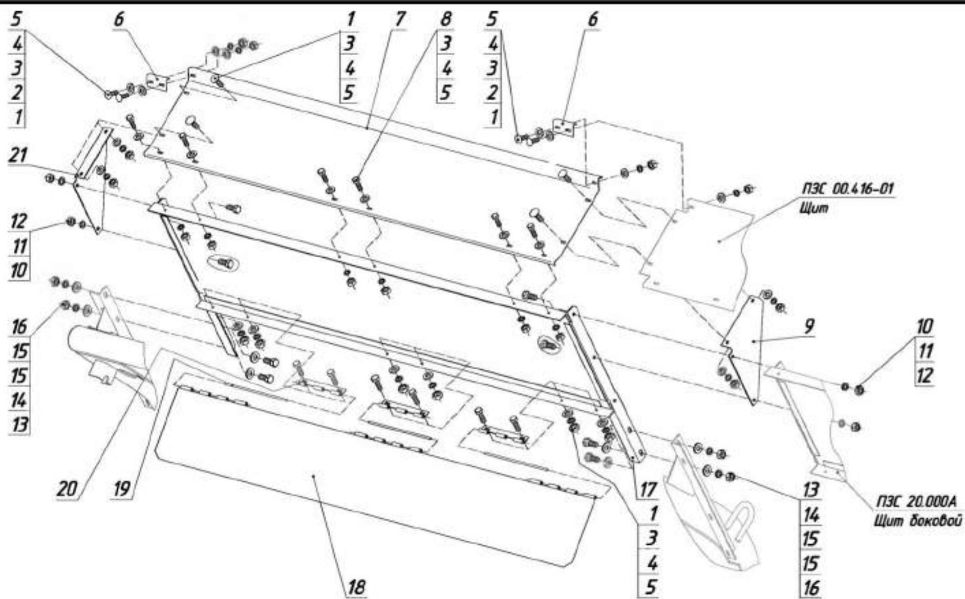
Корпус (левая сторона) (лист 1)
