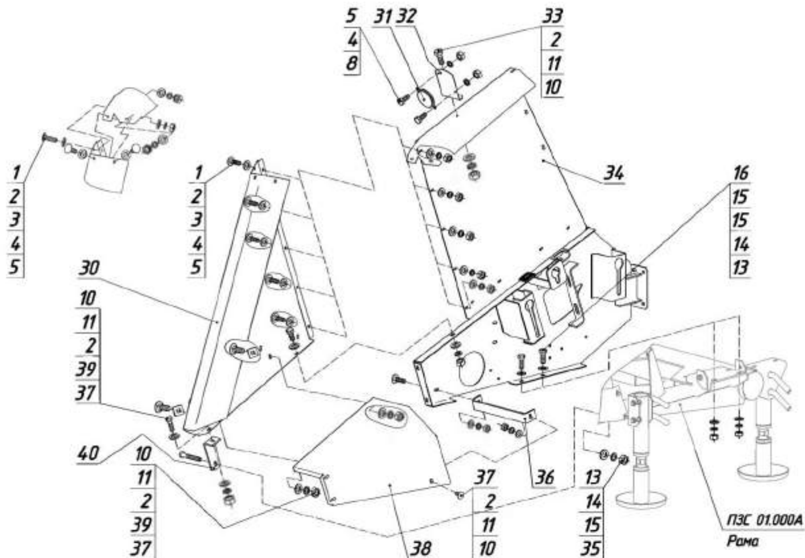
Корпус (левая сторона) (лист 3)
